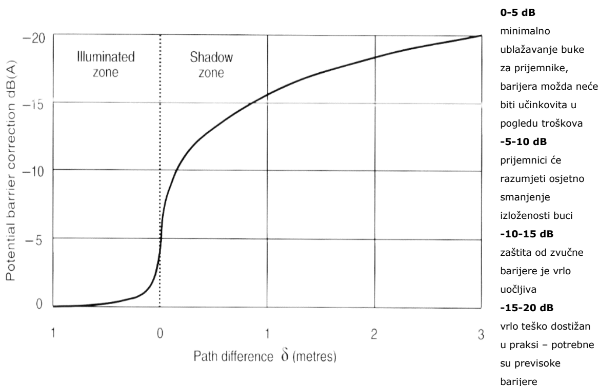
Slika 11-15: Bukobrani – Insercijski gubitak
