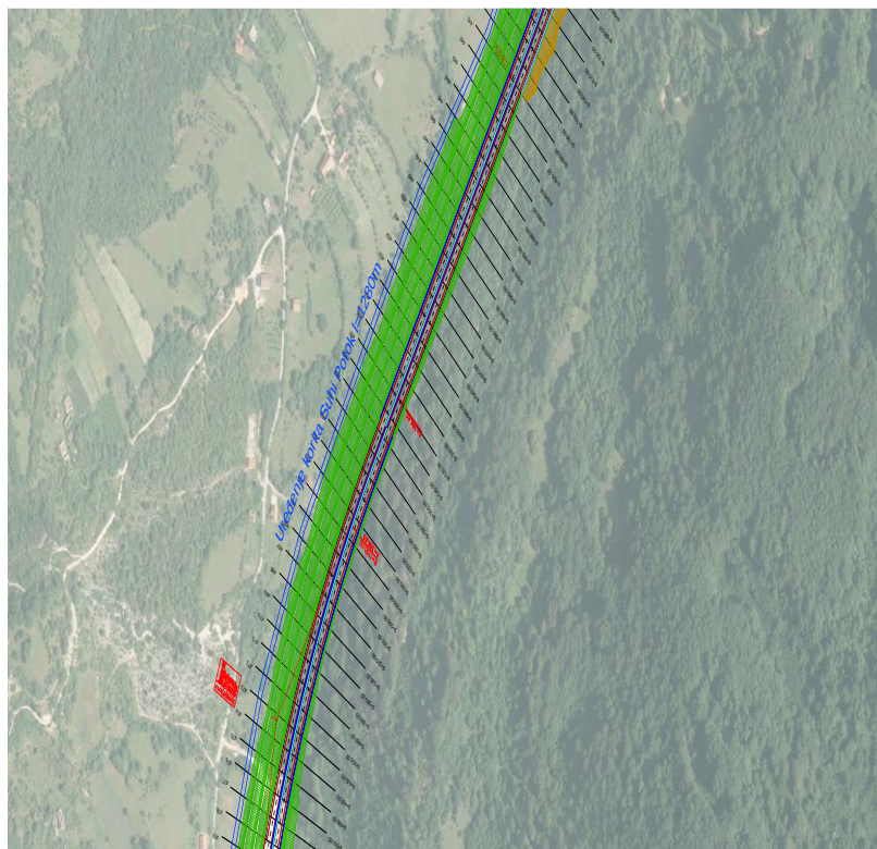
Slika 8-12: Regulacija vodotoka Suhog potoka ( L=1.280\text{ m} )
