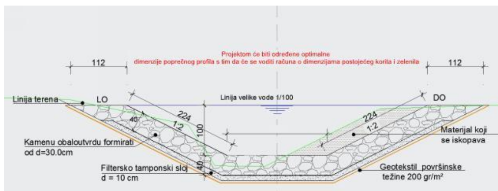
Slika 8-9: Regulacija rijeke Trešanice (L=140 m)
