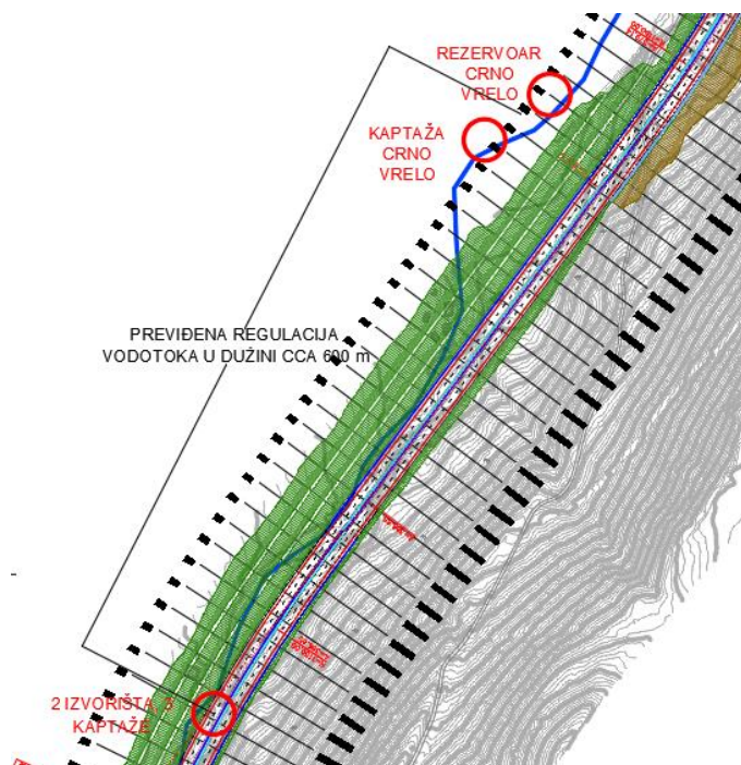
Slika 8-13: Regulacija vodotoka Bijela ( L= 600\text{ m} )
