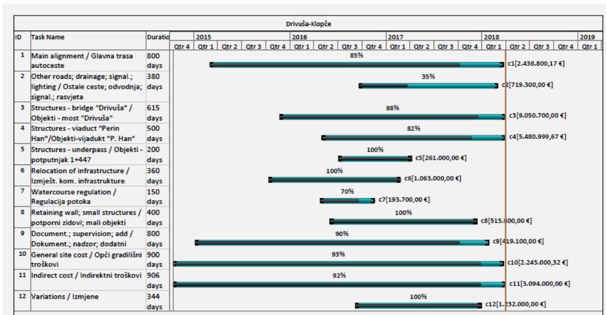
Gantogram 2. Prikazuje dinamiku građevinskih radova poddionica Drivuša - Klopče.
