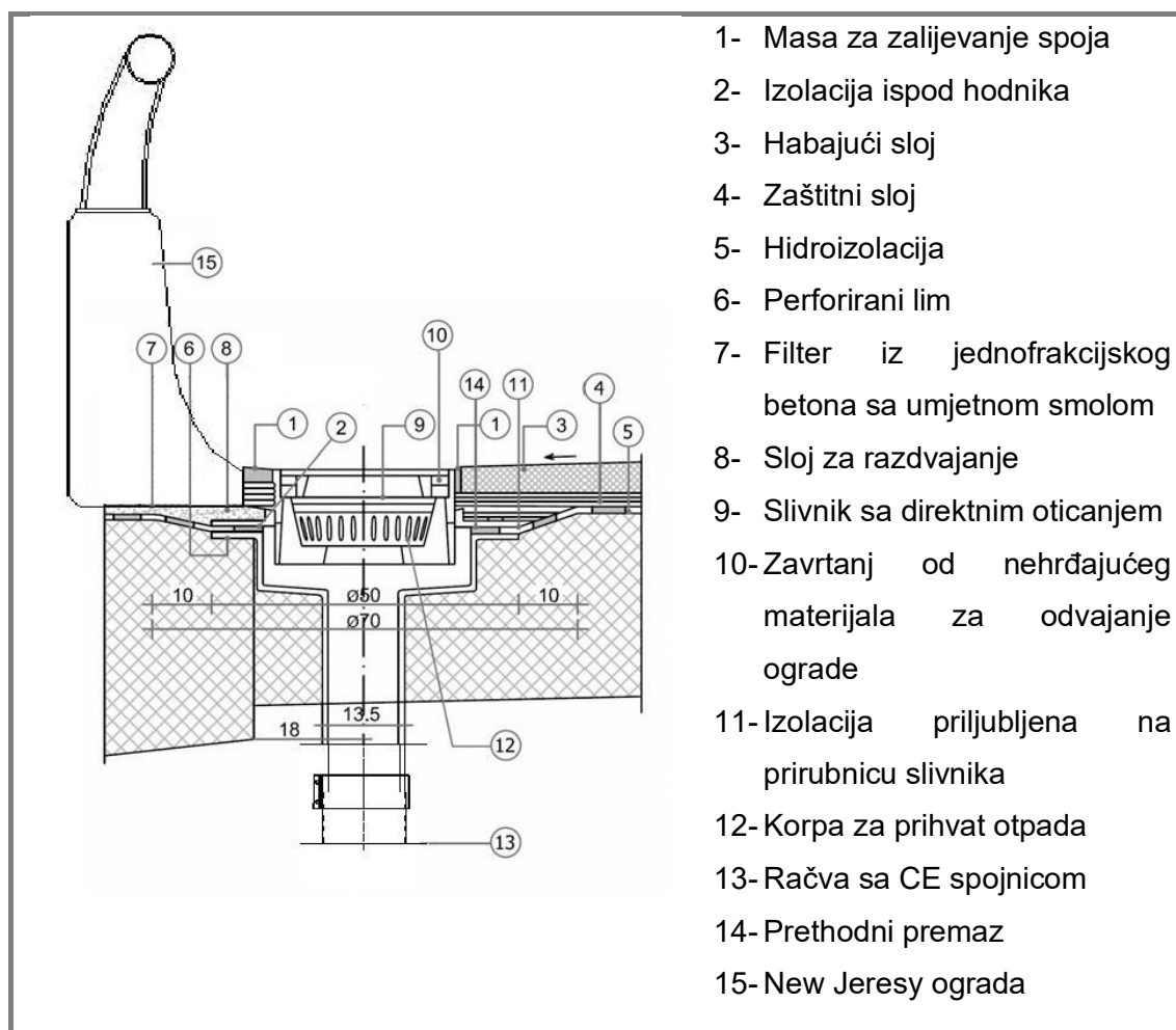
Slika 20: Detalj slivnika na objektu sa jendostranim nagibom i sa New Jersey ogradom
