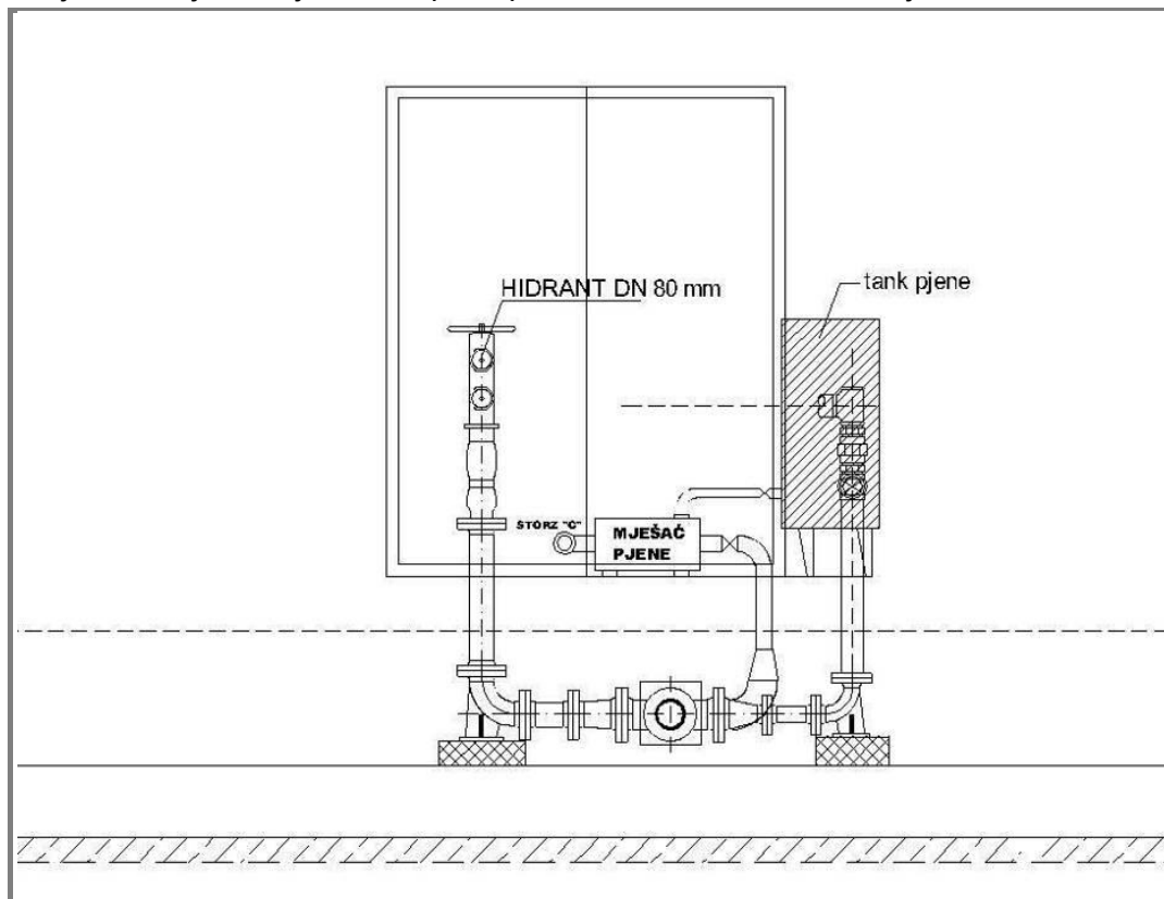
Slika 31: Detalj sistema protivpožarne zaštite u hidrantskoj niši
