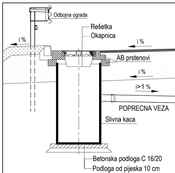
Slika 4: Detalj slivnika
