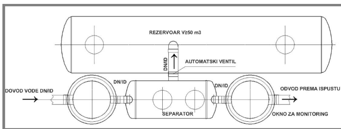
Slika 30: Šematski prikaz ispusta sistema iz centralnog sabirnog kolektora
