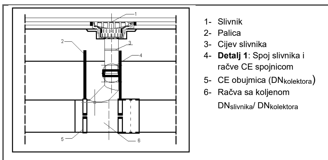
Slika 18: Spoj slivnika i račve na uzdužni kolektor na objektu Detalj spoja slivnika i račve CE spojnicom dat je na narednoj slici, kao i 3-D prikaz CE spojnice.
