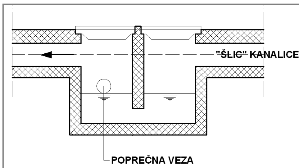
Slika 27: Detalj sifonskog šahta sa poprečnom vezom na centralni sabirni kolektor
