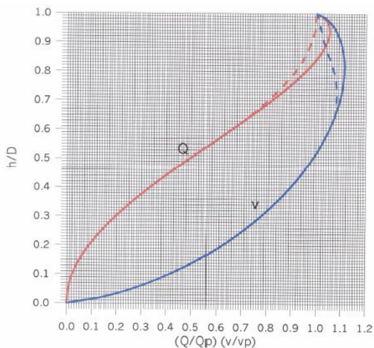
Slika 7: Zavisnost Q/Q_p i v/v_p od h/D za kružni profil cijevi
