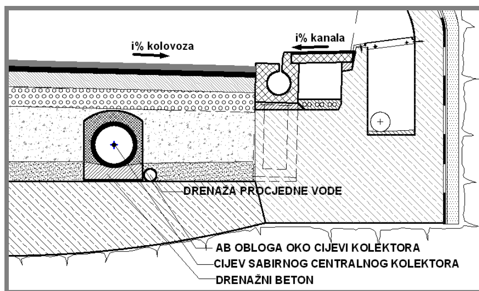
Slika 28: Detalj centralnog sabirnog kolektora u tunelu
