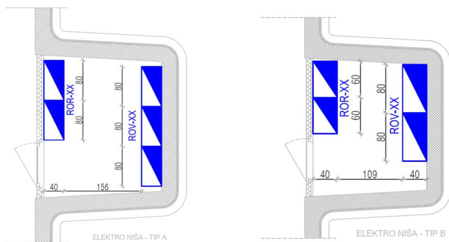
Slika 5 - Elektro niša - raspored opreme
