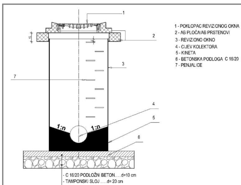
Slika 6: Detalj revizionog okna sa AB pločama/prstenovima
