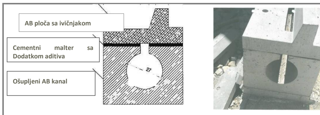
Slika 26: Prikaz kontinualne „šlic“ drenažne kanalice
