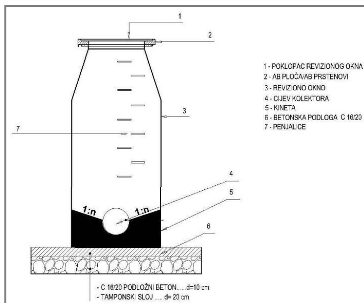
Slika 5: Detalj revizionog okna sa konusnim završetkom
